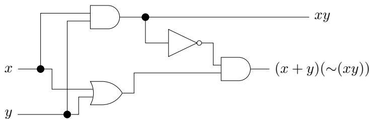
Abbildung 2.4.: Einfacherer Halbaddierer
